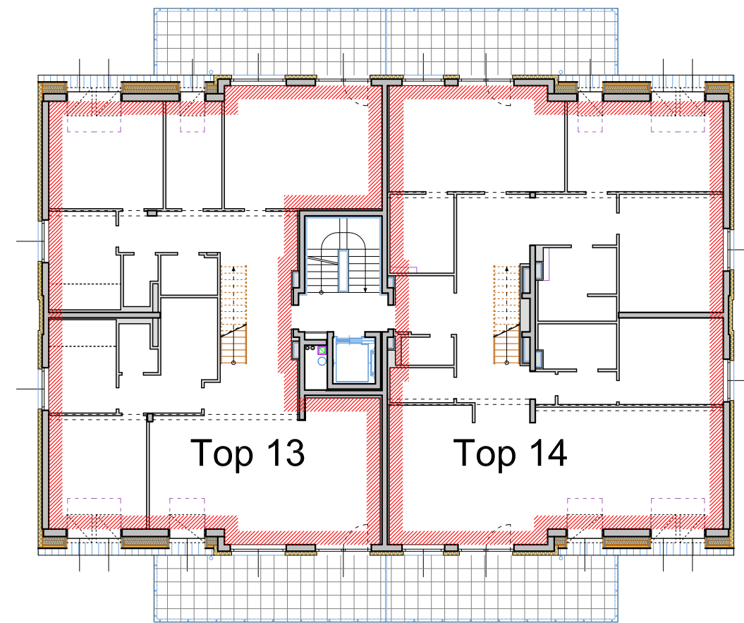
DACHGESCHOSS
