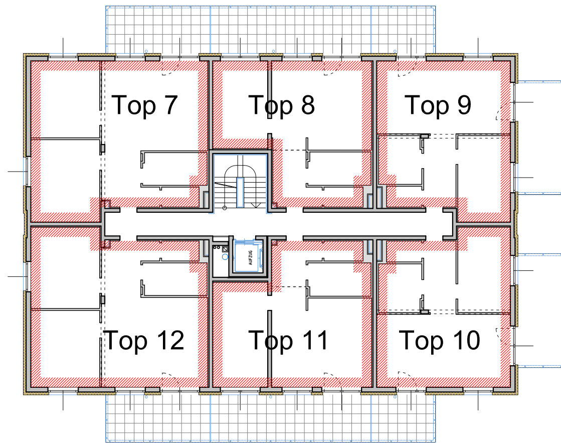
OBERGESCHOSS
