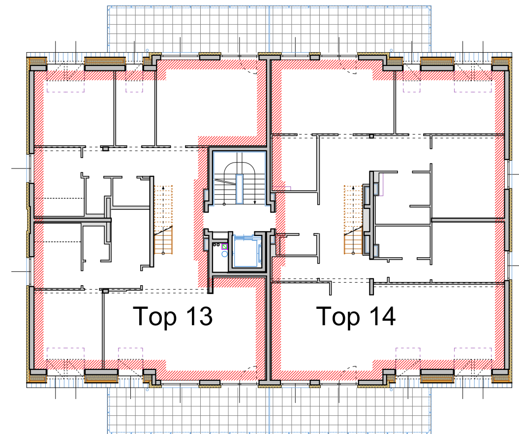
DACHGESCHOSS
